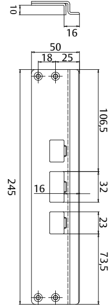
Mekaniskt slutbleck 547
